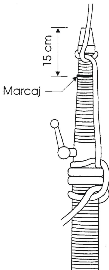
FIGURA c - FIXAREA ȚEVII CU CORDIȚA
